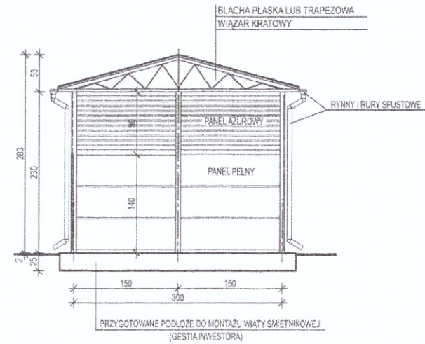
PRZEKRÓJ A - A 1:50
