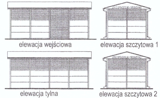
ELEWACJE 1:100
