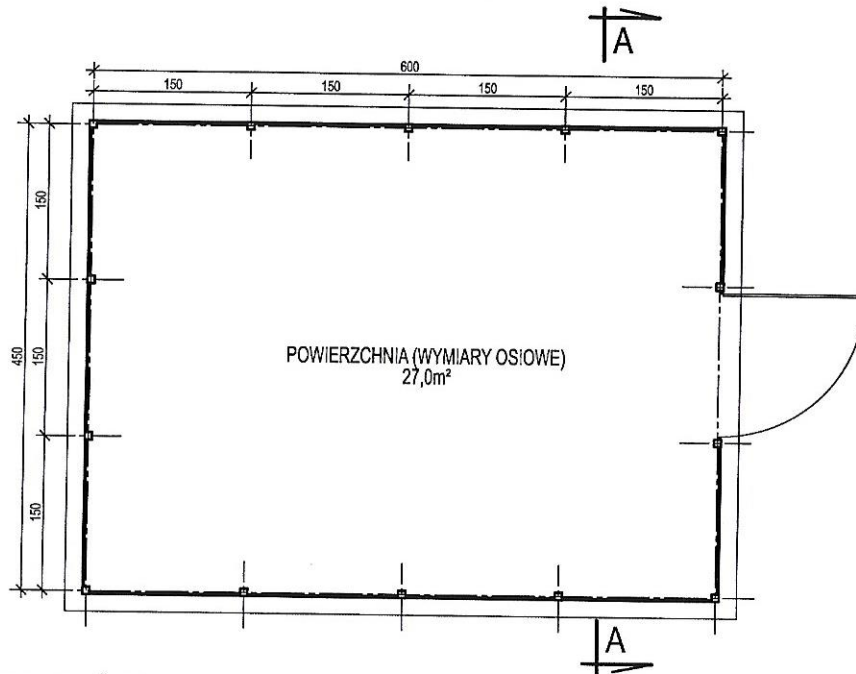
RZUT PRZYZIEMIA 1:50
