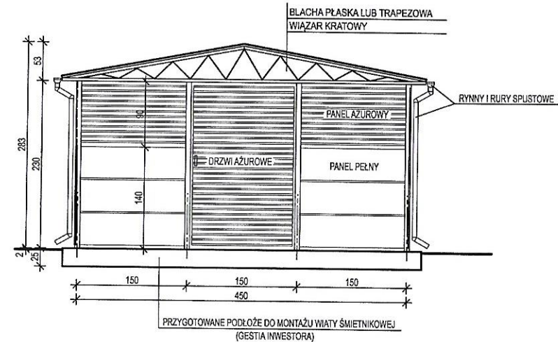
ELEWACJE 1:100
